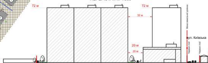
ПЕРЕРІЗ II-II. М 1:500
