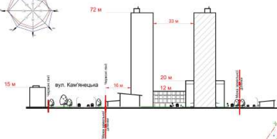
ПЕРЕРІЗ I-I. М 1:500
